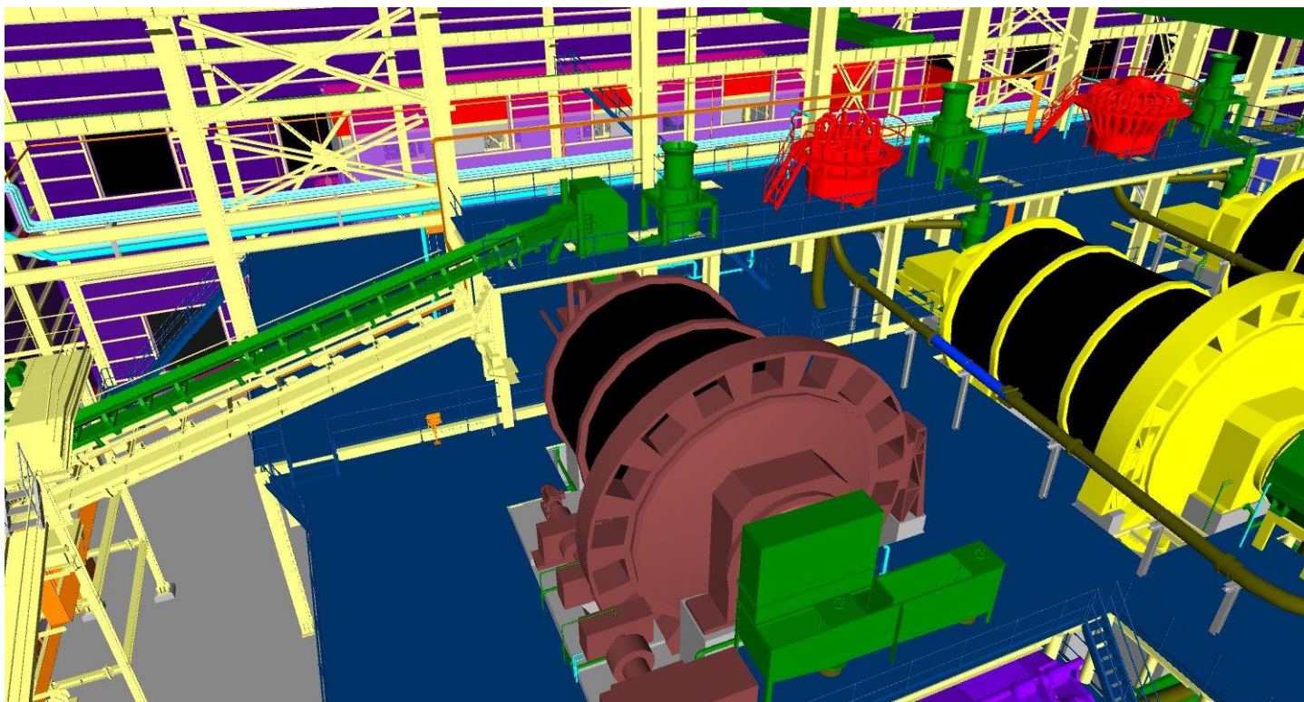
نمونه مدلسازی سه بعدی
